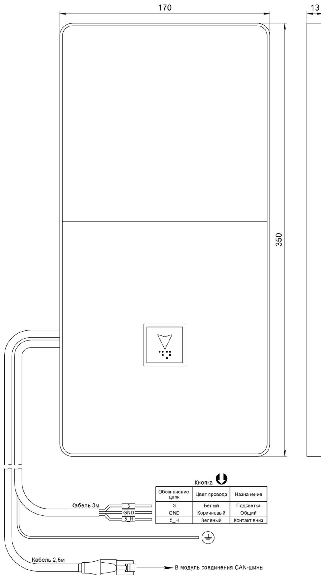
Рис.1 Внешний вид, габаритные и установочные размеры Вызывного поста МАЛАХИТ (жгут RJ45) НШЕК.468381.089
